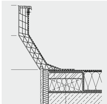
Eindichten Aufsetzkranz 3020
