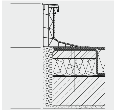
Eindichten Aufsetzkranz 1600
